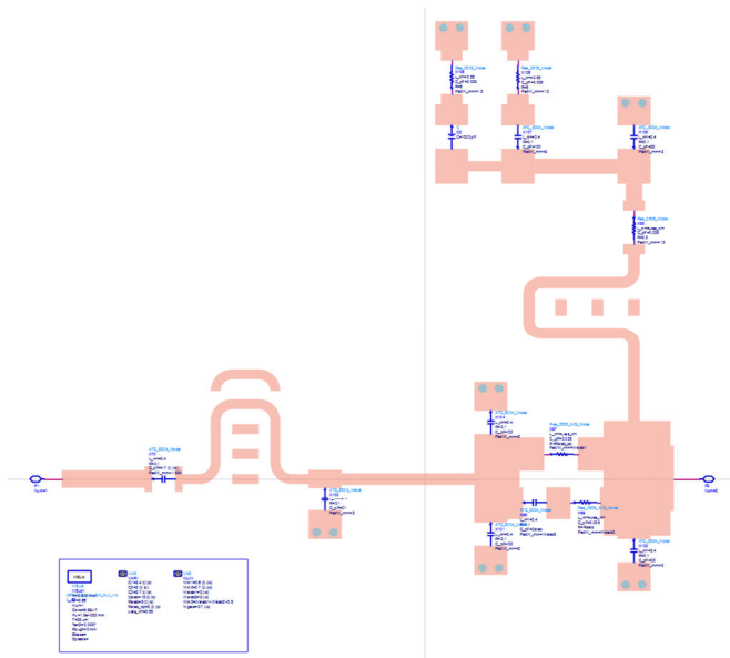
Figure 6: EM simulated input match
